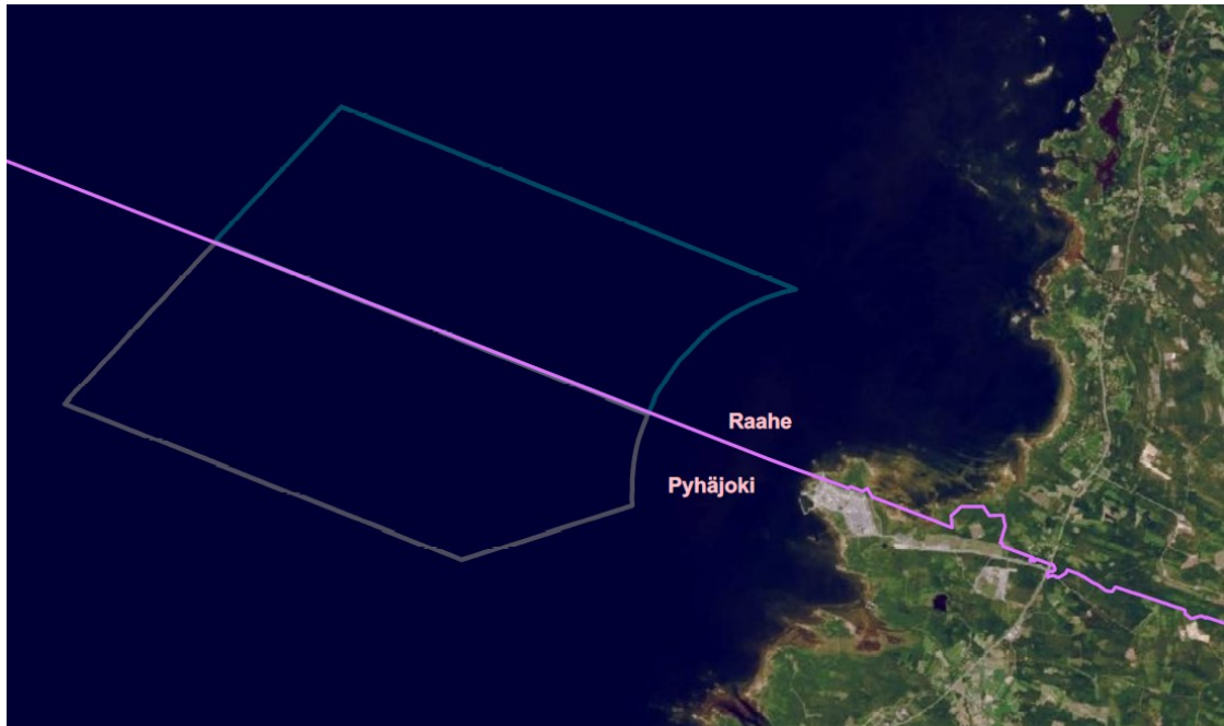
Kuva 8 Maanahkiaisien merituulivoimapaiston sijainti.
